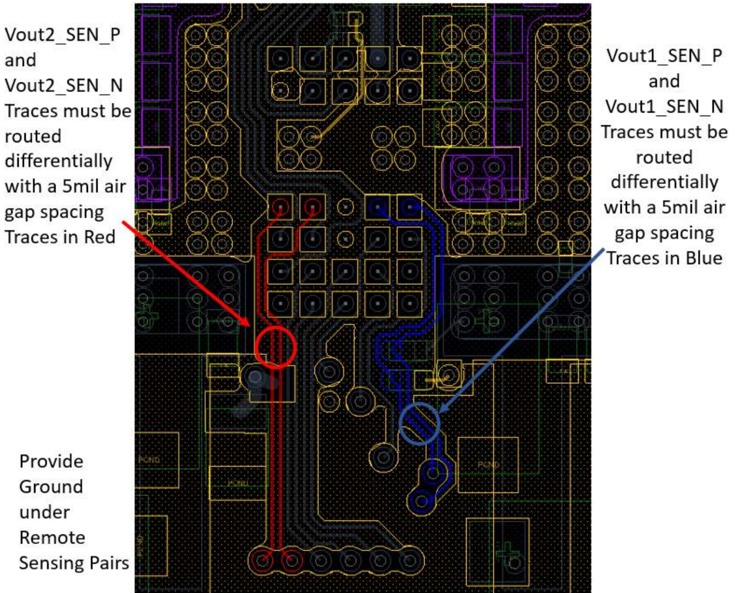
Figure 33 : VSense Traces
