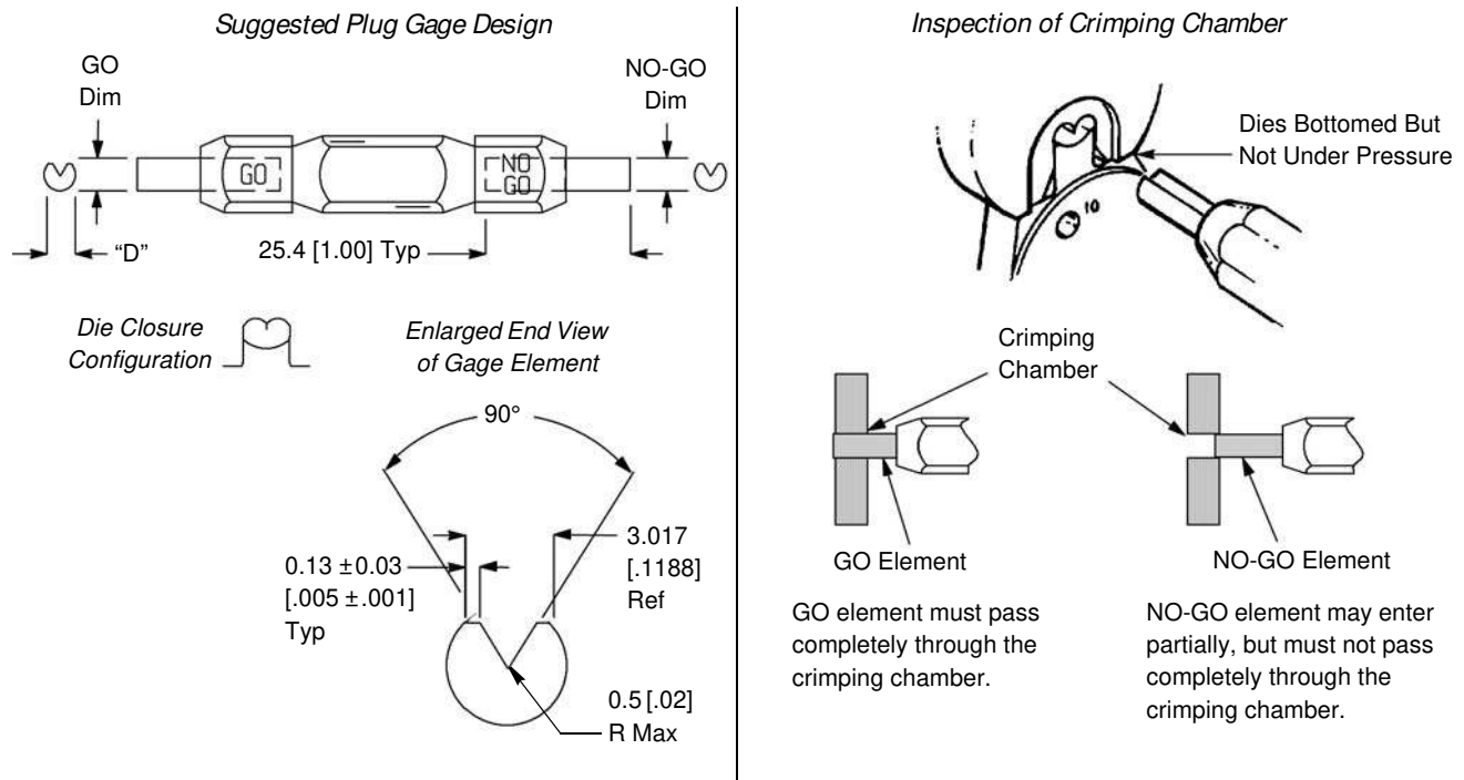
68321-1 F-CRIMP GAGE
