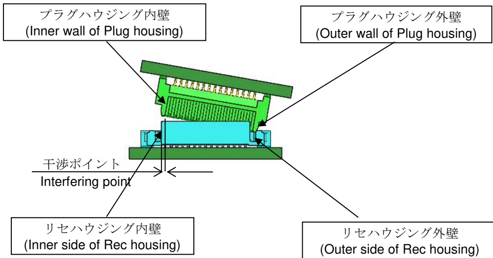
図-3 外壁合わせによる嵌合
