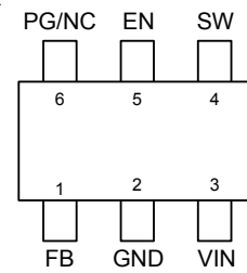
SOT-563 (FC)
