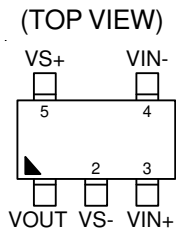
TSOT-23-5 RT9148
