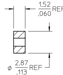
SPACER
