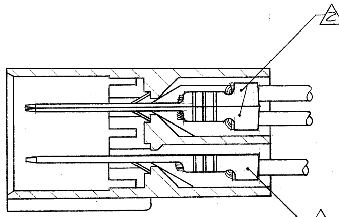
ファスティ-ファストンタブ接合状態 (FASTIN-FASTON TAB MATING STATE)
