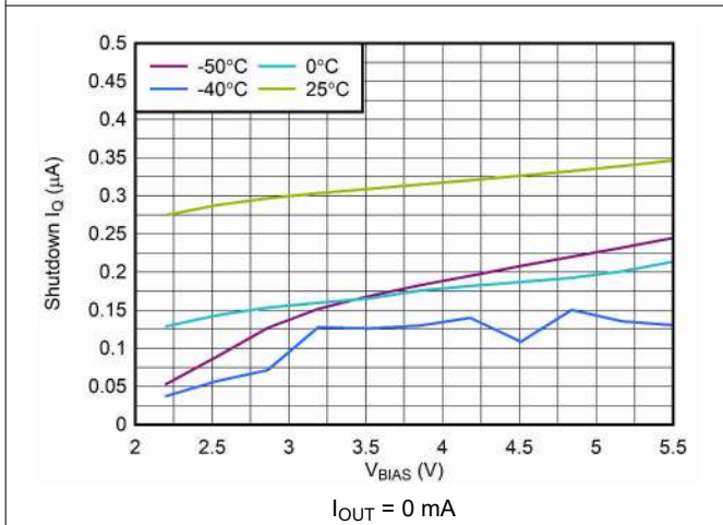
Figure 6-9. V_{\text{BIAS}} Shutdown I_Q vs V_{\text{BIAS}}
