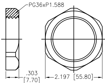
Ⓐ Lock Nut
