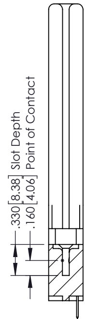
SECTION A-A
