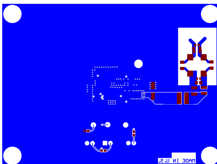
Figure 5-4. Bottom Layer
