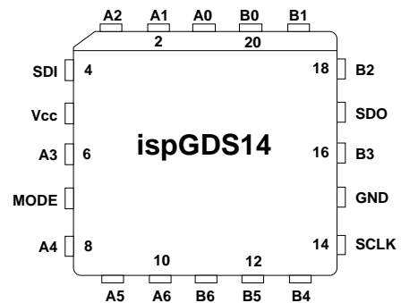
20-Pin PLCC
