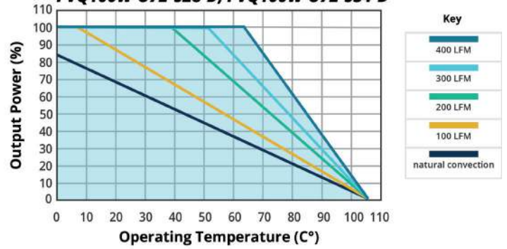
TEMPERATURE DERATING CURVE (Vin =72 V) PVQ100W-072-S15-D, PVQ100W-072-S24-D, PVQ100W-072-S28-D, PVQ100W-072-S54-D
