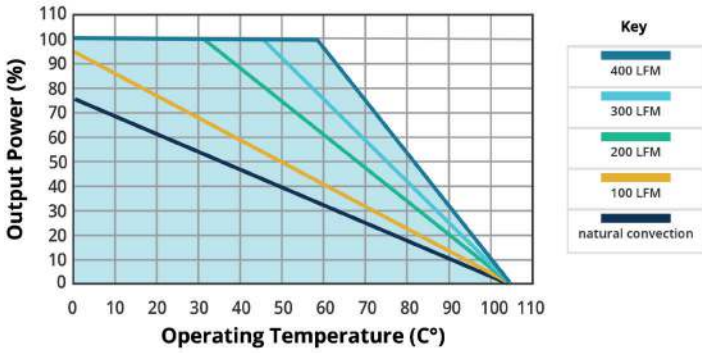
TEMPERATURE DERATING CURVE (Vin =72 V) PVQ100W-072-S5-D, PVQ100W-072-S12-D
