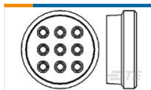
TE Part #HDC34-24-1E DUST CAP, 24SZ, PLG, AL, NO LANYARD,HD30
