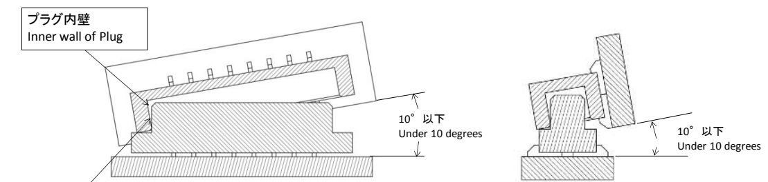
△ 図-2 内壁合わせによる嵌合 (Acceptable) Figure 2 Mating aligning to inner wall of housing
