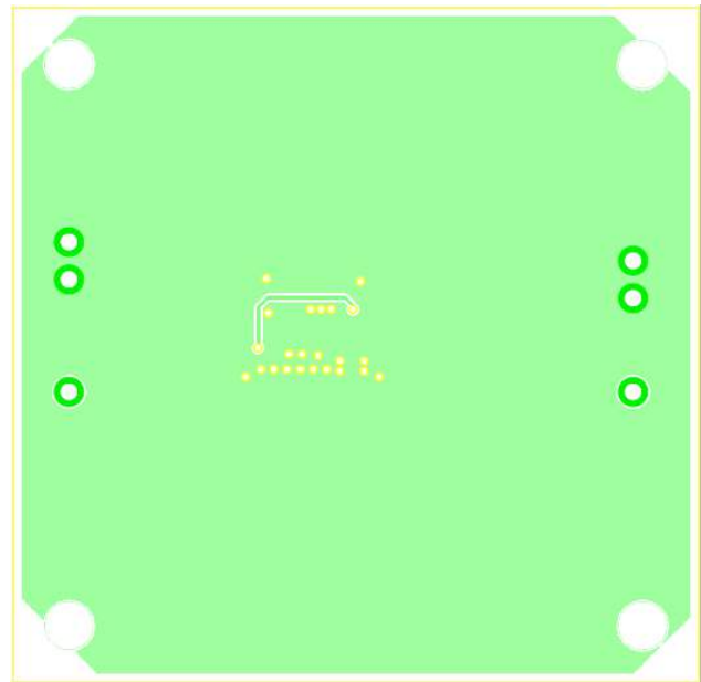
Figure 4—Bottom Layer
