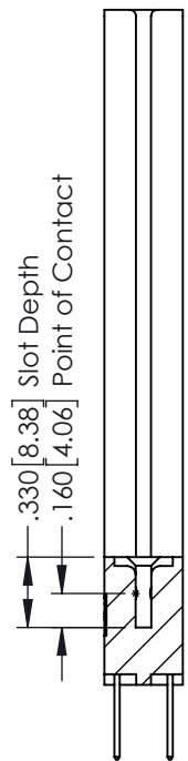
SECTION A-A
