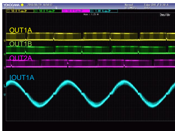
Figure 19. 1/16 STEP ( CLK : 9600Hz )
