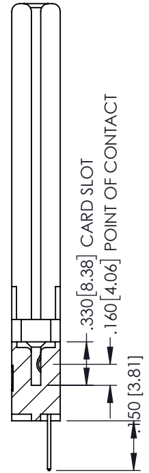
SECTION A-A
