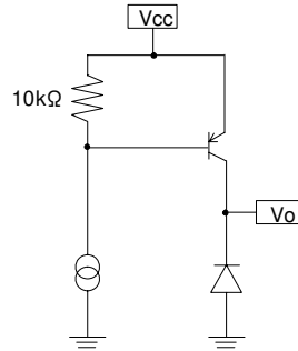
Vo Pin
