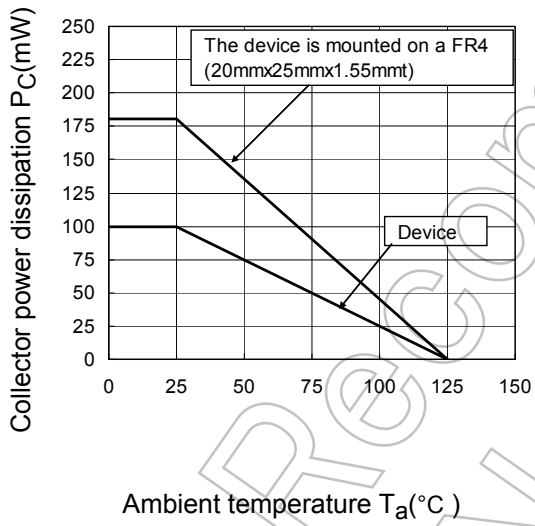
P_C - T_a
