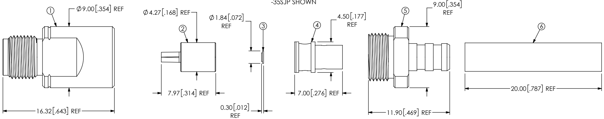
FIG 6 -35SJP SHOWN
