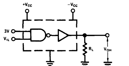
FIGURE 2. V IL , V OH
