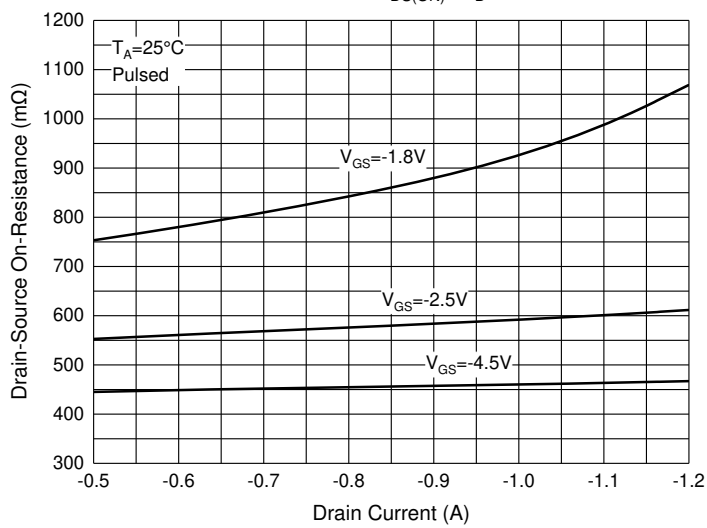
Fig. 3 - R_{DS(ON)} - I_D
