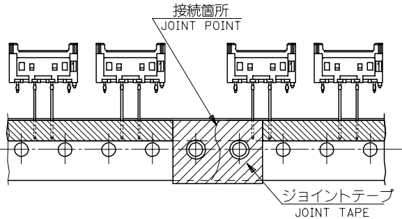
極数別テーピング状態図 CKT.TAPING FORM
