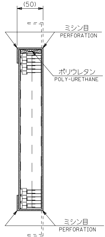
竹串 BAMBOO SKEWERS 包装状態図 PACKAGING FORM
