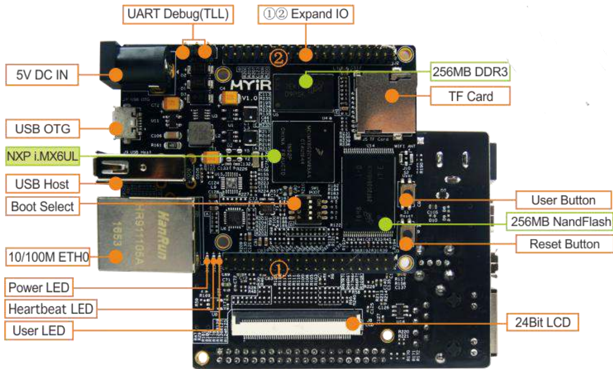
MYS-6ULX-IND
