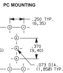
E101J1_BE2 SPDT
