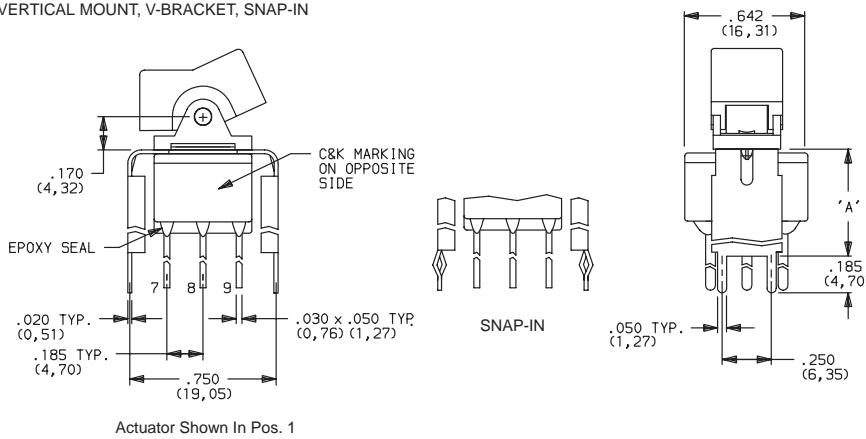
E301J1__BE2 3PDT
