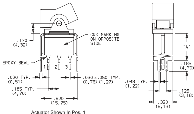
E101J1V3BE2 SPDT
