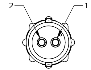
WIRING VIEW W18280-2SG-P-3XX
