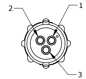
WIRING VIEW W18280-3SG-P-3XX
