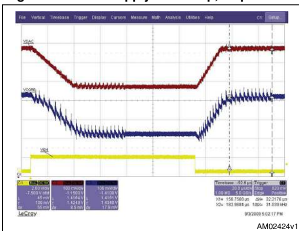
Figure 27. GFX supply - VID step, skip mode
