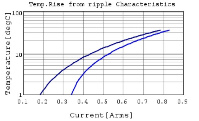
GJM0335C1E1R5CB01 Temp.rise — 3GHz — 4
