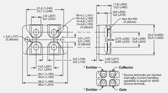
SOT-227
