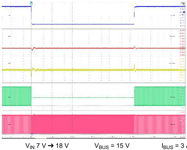
V_{IN} = 7\text{ V} \rightarrow 18\text{ V} V_{BUS} = 15\text{ V} I_{BUS} = 3\text{ A} Figure 10-36. Line Transient: V_{BUS} = 15\text{ V}
