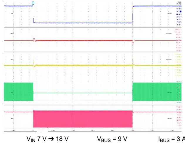
V_{IN} = 7\text{ V} \rightarrow 18\text{ V} V_{BUS} = 9\text{ V} I_{BUS} = 3\text{ A} Figure 10-37. Line Transient: V_{BUS} = 9\text{ V}
