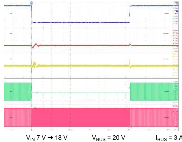
V_{IN} = 7\text{ V} \rightarrow 18\text{ V} V_{BUS} = 20\text{ V} I_{BUS} = 3\text{ A} Figure 10-35. Line Transient: V_{BUS} = 20\text{ V}
