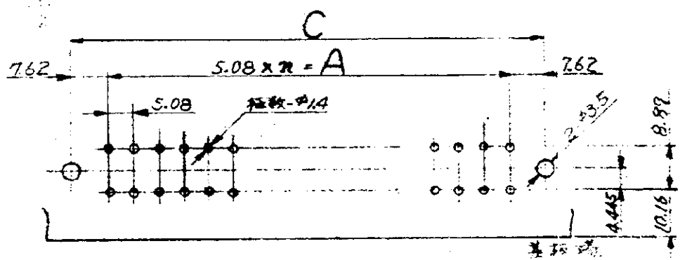
基板推奨穴位置 (基準原 2-762)
