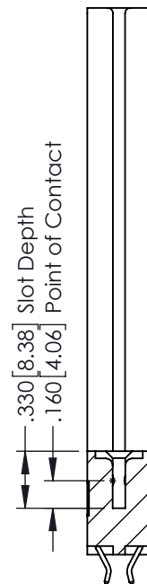
SECTION A-A
