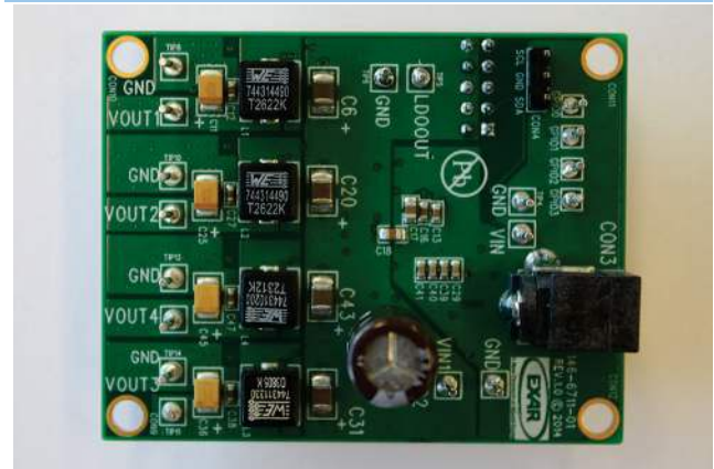
XRP7714EVB-DEMO-3
