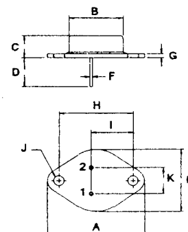
TO-3
