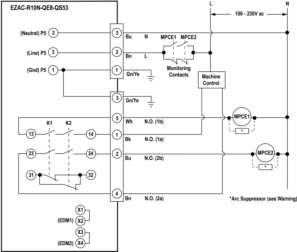
Figure 11. Wiring—model EZAC-R10N-QE8-QS53
