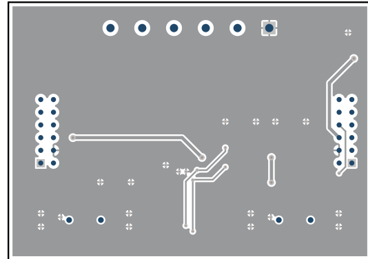
Figure 6-8. SENS063 Bottom Layer
