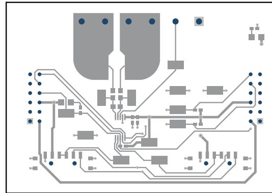
Figure 6-6. SENS063 Top Layer
