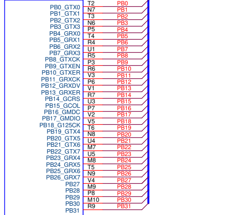
MN2B SAMA5D3x BGA324
