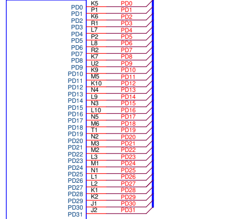
MN2D SAMA5D3x BGA324
