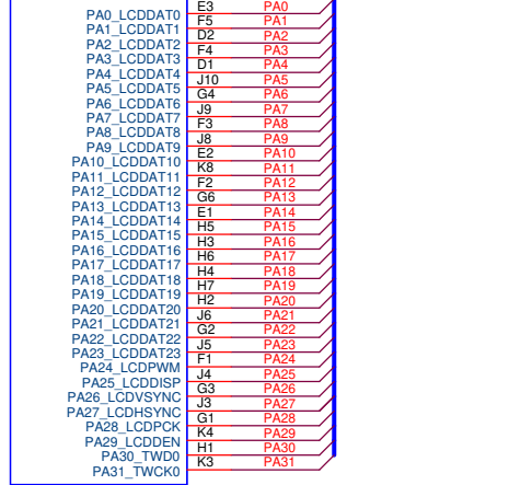
MN2A SAMA5D3x BGA324
