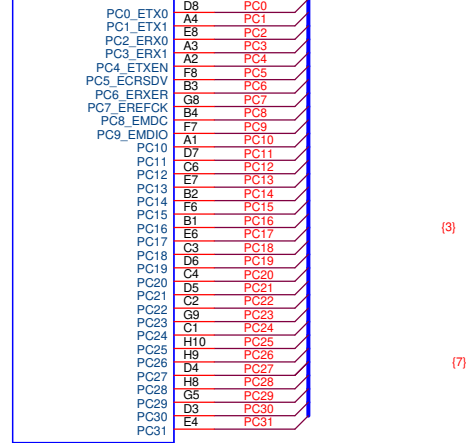
MN2C SAMA5D3x BGA324
