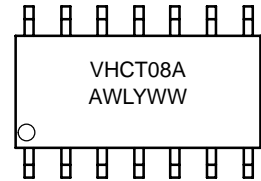
SOIC-14 D SUFFIX CASE 751A
