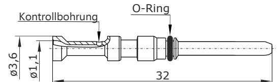
Hauptabmessungen Kontaktstift
