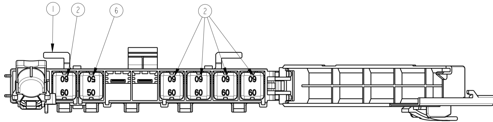
TE PN FORD PN 1380296-8 6S65-14517-DB SCALE 1:1
