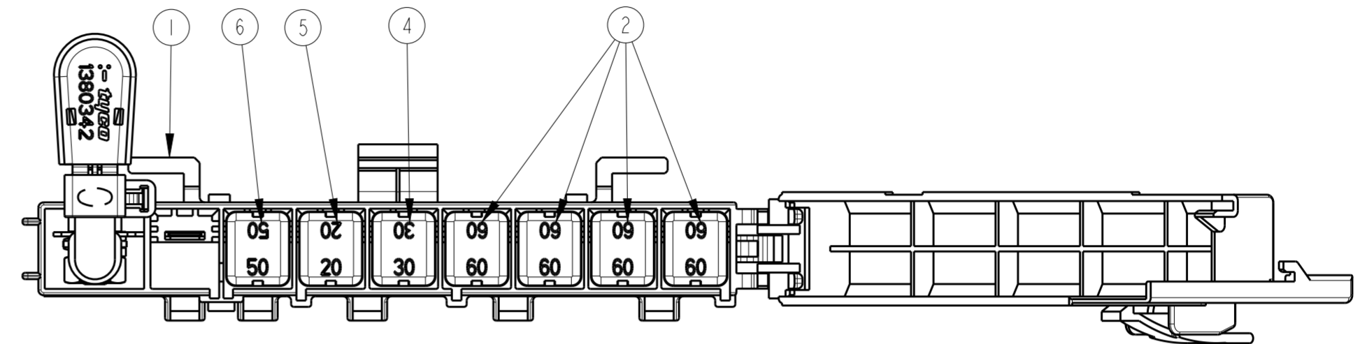
TE PN FORD PN 1380296-7 6S65-14517-CA SCALE 1:1
