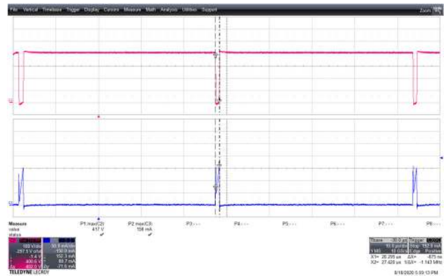
Figure 33 – 300 VAC 60 Hz. CH2: V_{DS} , 100 V / div., 10 \mu s / div. CH3: I_{DS} , 50 mA / div., 10 \mu s / div. V_{DS(MAX)} = 417 V. I_{DS(MAX)} = 158 mA.
