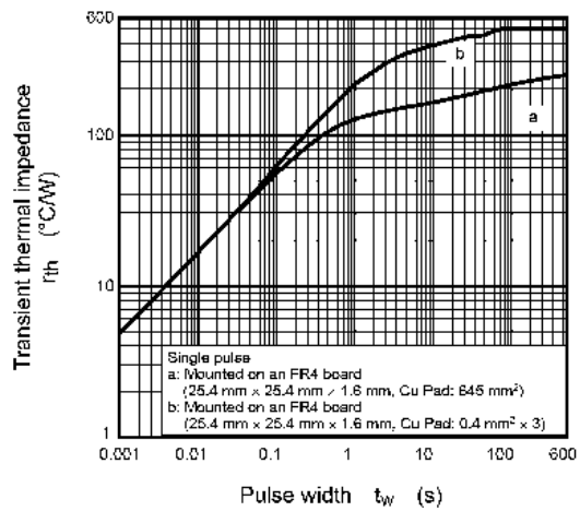
Fig. 8.12 r_{th} - t_w
