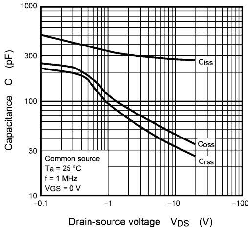
Fig. 8.9 C - V_{DS}
