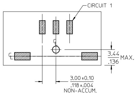
3 CKT CONFIGURATION
