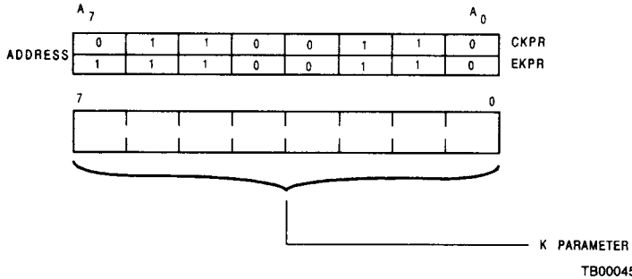
Figure 28. K Parameter Registers (CKPR, EKPR)
