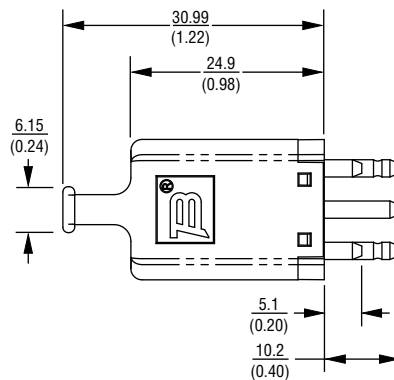
2410-7 MODULE
