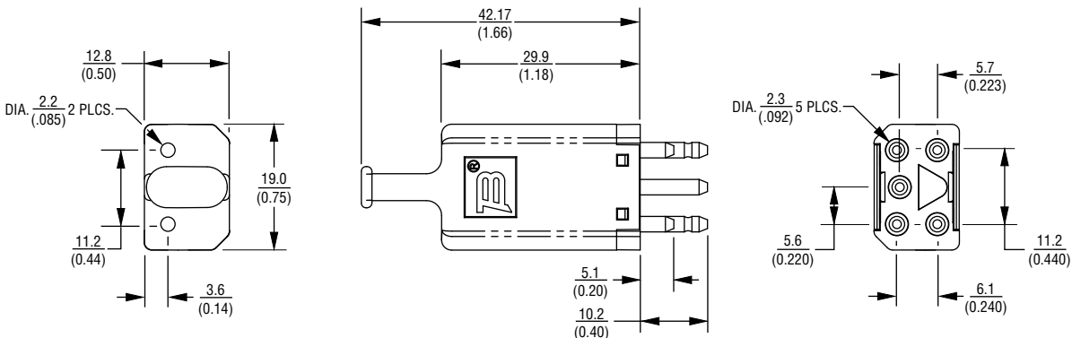
2410-3 MODULE
