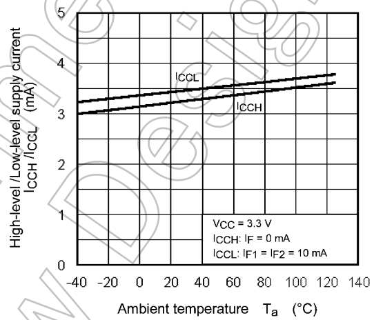
Fig. 12.2.10 I_{CCH}/I_{CCL} - T_a
