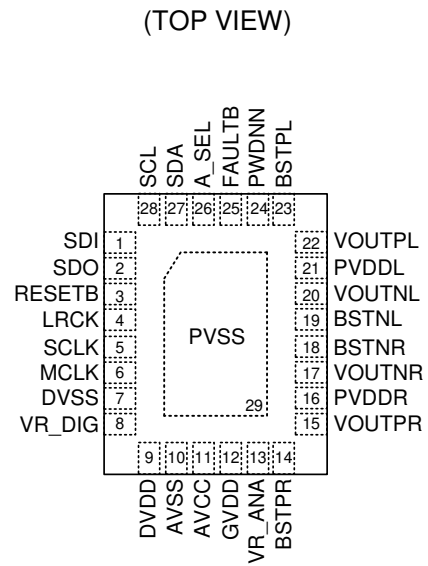
VQFN-28L 4x5
