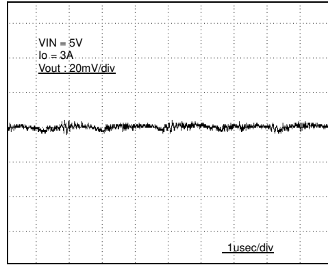
Fig.12 Output ripple
